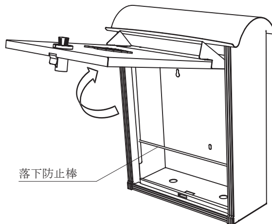
取出時 取出口サイズ 260 mm × 310 mm
