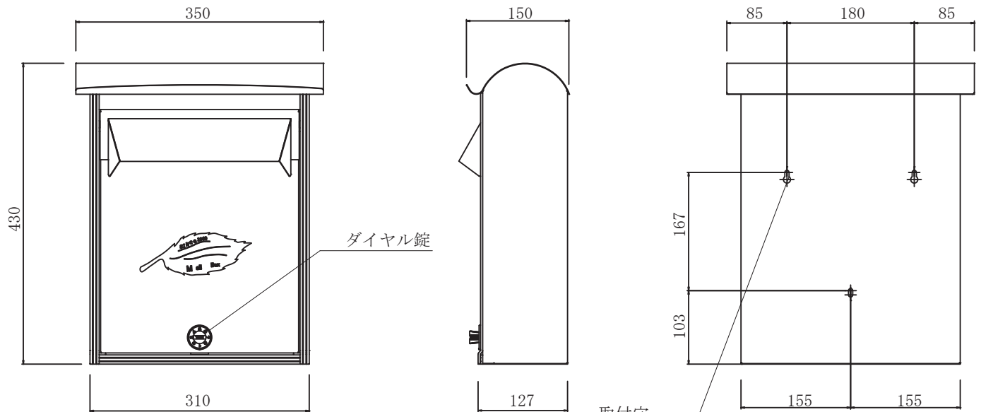
図は NL1-P18 ポスト底面にロットナンバーを記載
